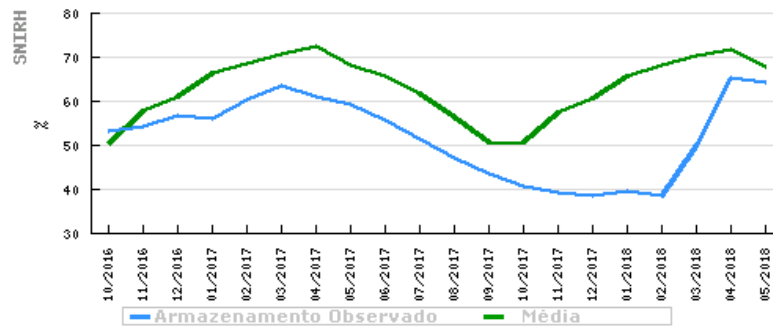
Figura 21 – Evolução dos volumes armazenados na bacia hidrográfica das Ribeiras do Oeste comparativamente à média mensal calculada para o período (1990/91 a 2016/17) (Fonte: APA).
