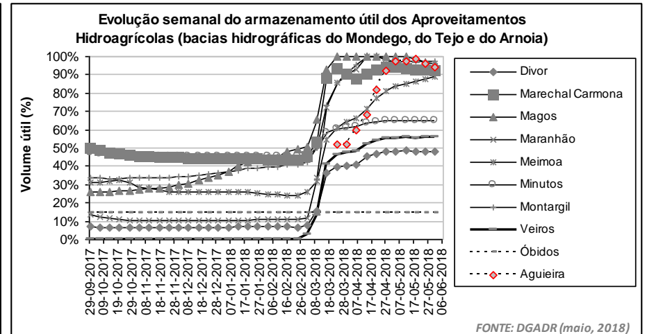
Figura 25 - Evolução semanal percentual dos volumes armazenados úteis dos aproveitamentos hidroagrícola das bacias hidrográficas do Douro e Vouga; Mondego, Tejo e Arnoia; Sado e Mira; Guadiana e ribeiras do Algarve.
