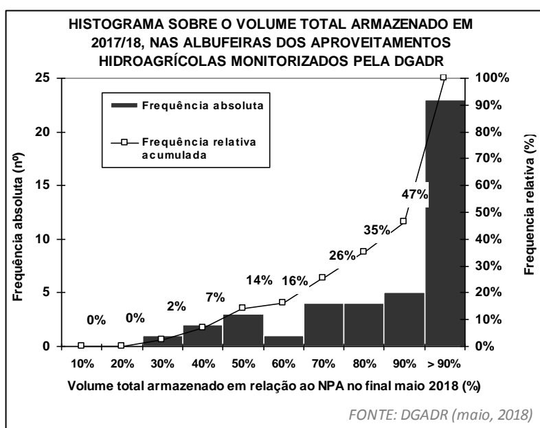
Figura 24- Histograma do volume total armazenado nas albufeiras dos aproveitamentos hidroagrícolas em maio de 2018 (Fonte: DGADR).
